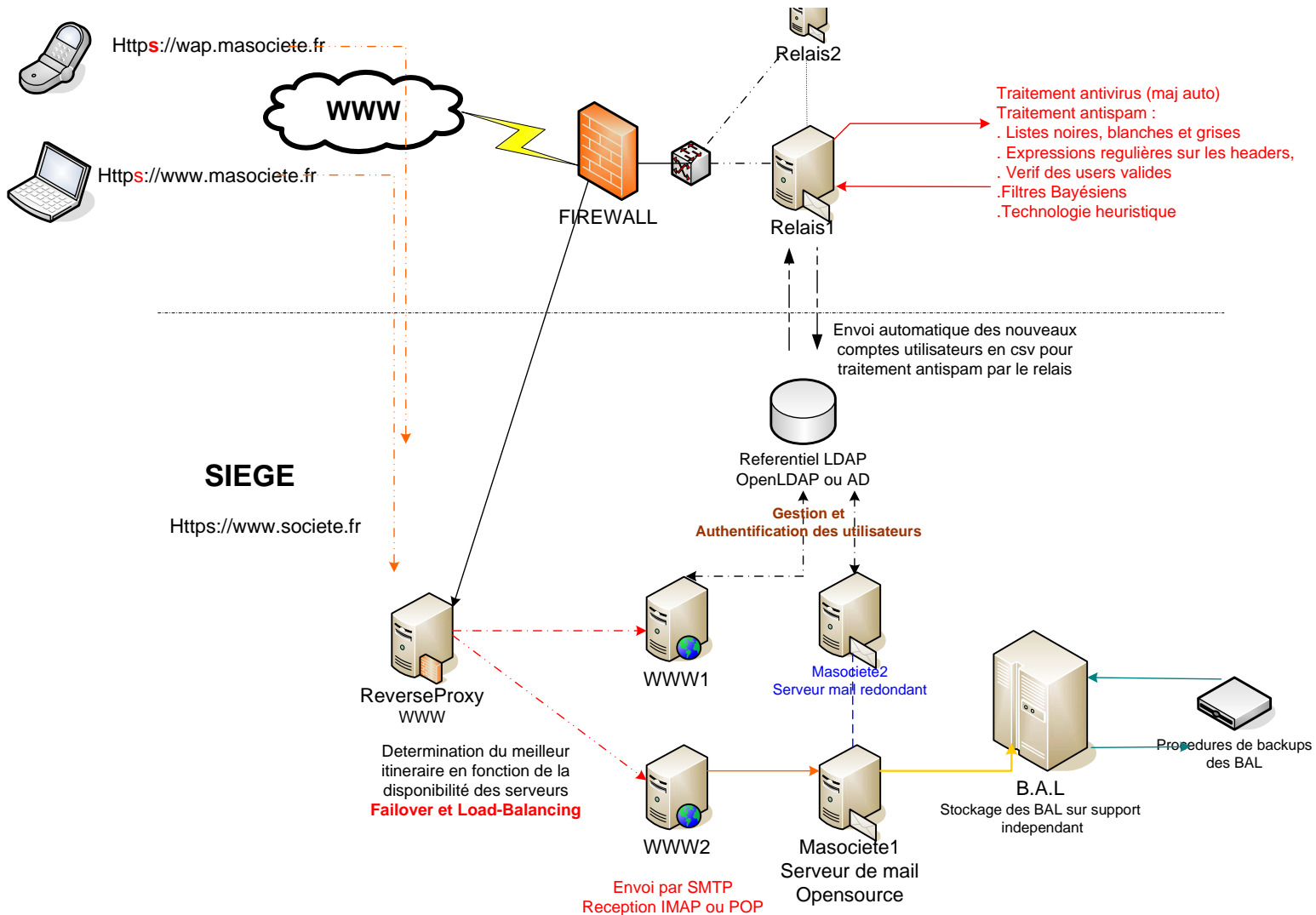
[exemple schéma d'architecture - relais + messagerie]
